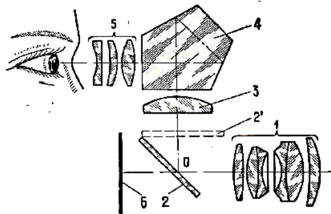
Рис. 1. Оптическая схема видоискателя
