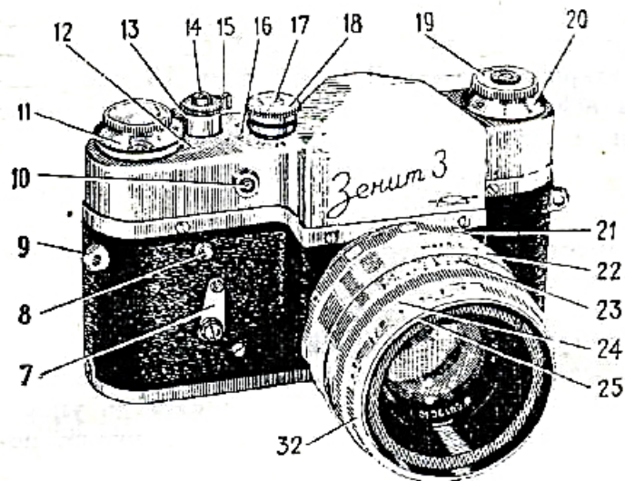
Рис. 2. Фотоаппарат «Зенит-3»
