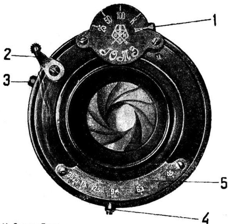
11. Затвор «Гомз».
