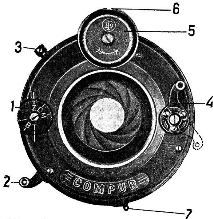
9. Затвор «Компур».
