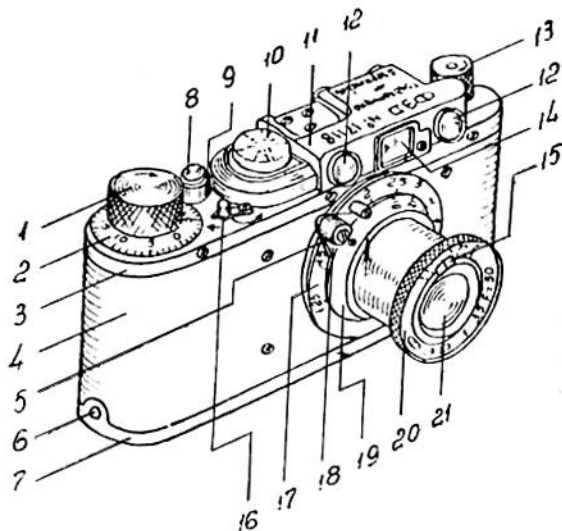
Рис. 1. Общий вид аппарата „ФЭД“ и детали механизма управления аппаратом. 1) Головка затвора. 2) Шкала счетчика кадров. 3) Верхняя (несъемная) крышка. 4) Корпус. 5) Кнопка рычажка червячного хода. 6) Стержень. 7) Нижняя (съемная) крышка. 8) Кнопка-спуск. 9) Кольцо с резьбой кнопки. 10) Шкала скоростей. 11) Корпус оптических видоискателя и дальномера. 12) Линзы оптического дальномера. 13) Головка для перематывания пленки. 14) Линза оптического видоискателя. 15) Движок шкалы диафрагмы. 16) Выключатель подачи пленки. 17) Шкала расстояний. 18) Рычажок червячного хода. 19) Шкала глубины резкости. 20) Переднее кольцо оправы объектива со шкалой диафрагмы. 21) Об'ектив.
