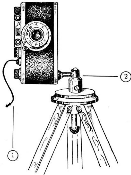
Рис. 16. Положение аппарата при съемке со штатива на вертикальный формат. 1) Проводочный трос. 2) Штативная головка.
