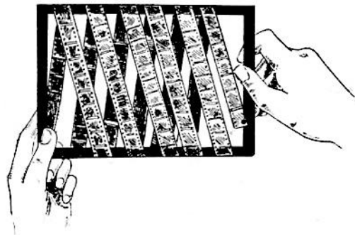
Рис. 18. Проявительная рамка с намотанной на нее пленкой.
