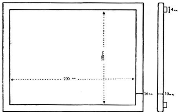
Рис. 17. Размерный чертеж рамки для проявления пленки.
