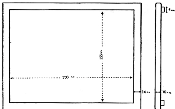
Рис. 17. Размерный чертеж рамочки для проявления пленки.
