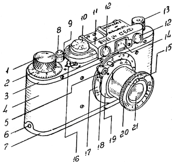
Рис. 1. Общий вид аппарата „ФЭД“ и детали механизма управления аппаратом. 1) Головка затвора. 2) Шкала счетчика кадров. 3) Верхняя (нес'емная) крышка. 4) Корпус. 5) Кнопка рычажка червячного хода. 6) Стержень. 7) Нижняя (с'емная) крышка. 8) Кнопка-спуск. 9) Кольцо с резьбой кнопки. 10) Шкала скоростей. 11) Корпусе оптических видоискателя и дальномера. 12) Линзы оптического дальномера. 13) Головка для перематывания пленки. 14) Линза оптического видоискателя. 15) Движок шкалы диафрагмы. 16) Выключатель подачи пленки. 17) Шкала расстояний. 18) Рычажок червячного хода. 19) Шкала глубины резкости. 20) Переднее кольцо оправы объектива со шкалой диафрагмы. 21) Объектив.
